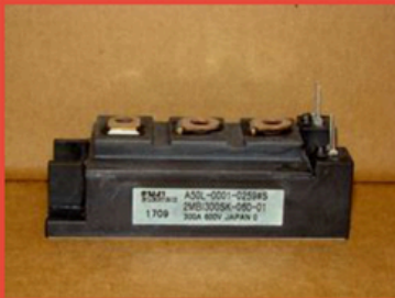
2MBI300SK- 060- 01
